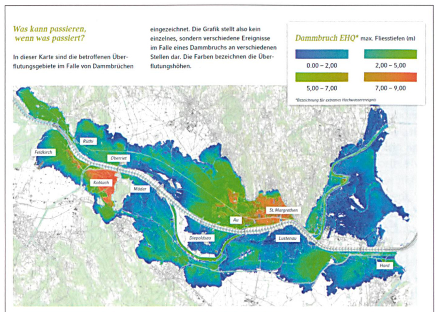
Abb. 7: Dammbüch Überflutungskarte EHQ (entspricht HQ300).
