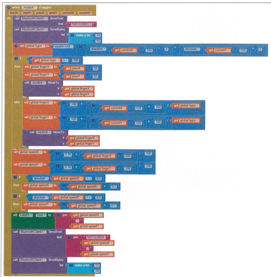
Abb. 3: Quellcode.
