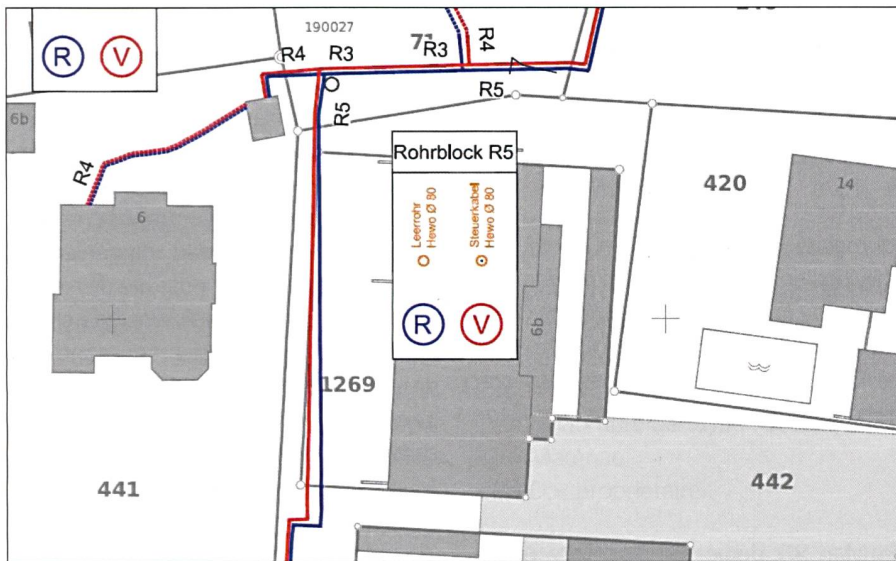
Abb. 2: Planausschnitt aus bestehendem Werkplan 4207.1, Schmalz Ing. AG. Fig. 2: Extrait de l'actuel plan d'ouvrage 4207.1, Schmalz Ing. AG. Fig. 2: Estratto del piano esistente dell'opera 4207.1, Schmalz Ing. AG.
