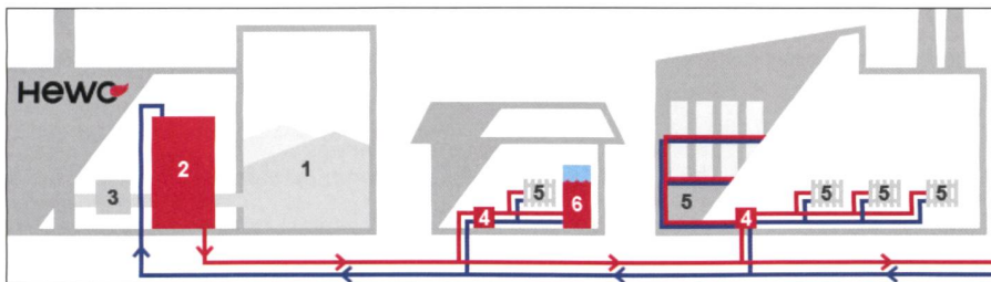
Abb. 1: Wärmekreislauf 2 .
