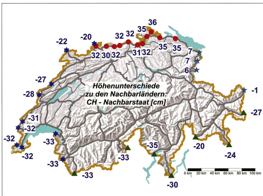
Abb. 3: Höhenunterschiede an der Landesgrenze in [cm].
