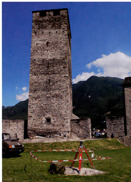
Abb. 2: GNSS-Landesnetz LV95. Stationierung auf Verdichtungspunkt «Bellinzona» (Castelgrande) in der Messkampagne CHTRF2010 (Foto swisstopo).
