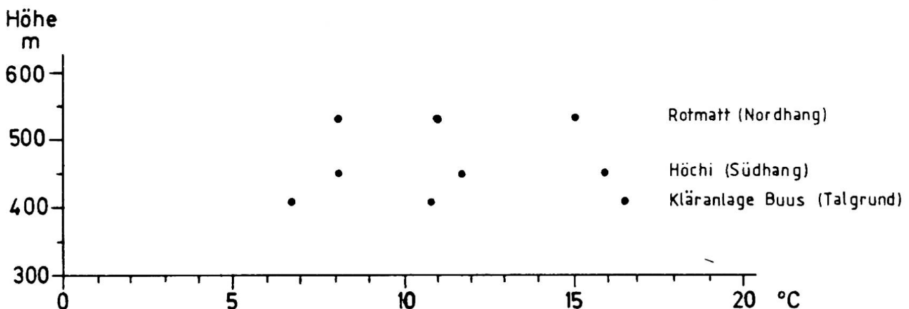
Fig. 2 Tägliche Minima, Mittel und Maxima der Temperatur an einem Nordhang, Südhang und im Talgrund (Mittelwerte der Jahre 1963–80 für die Monate März bis November)
