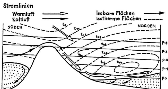
Abb. 5 Das zyklonale Hauptstadium einer Süd föhnlage. Die Föhnströmung vermag bis in die Täler hinunter vorzudringen. Diese Entwicklung wird ermöglicht durch den großen Druckgradienten und das gut entwickelte Solenoidfeld, die der Föhnströmung auf der Leeseite die notwendige Absinkbeschleunigung und Energie verschaffen.
