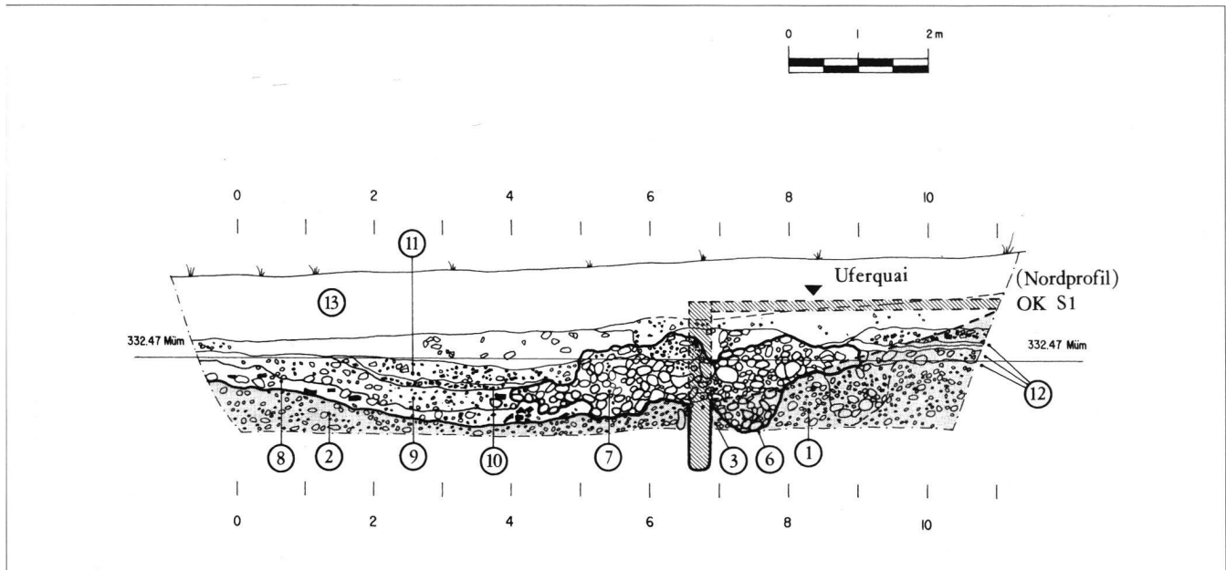
Abb. 5: Windisch-Spitzmatt. Westprofil mit Schnitt durch die rekonstruierte Uferbefestigung und Verlauf der älteren Uferböschung auf natürlich anstehendem Flussskies S1 mit römischen Funden vermishtem Flusssediment S2 (grau, Zeichnung C. Wesp).
