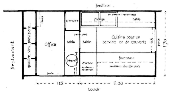
Plan d'une cuisine de wagon-restaurant.
