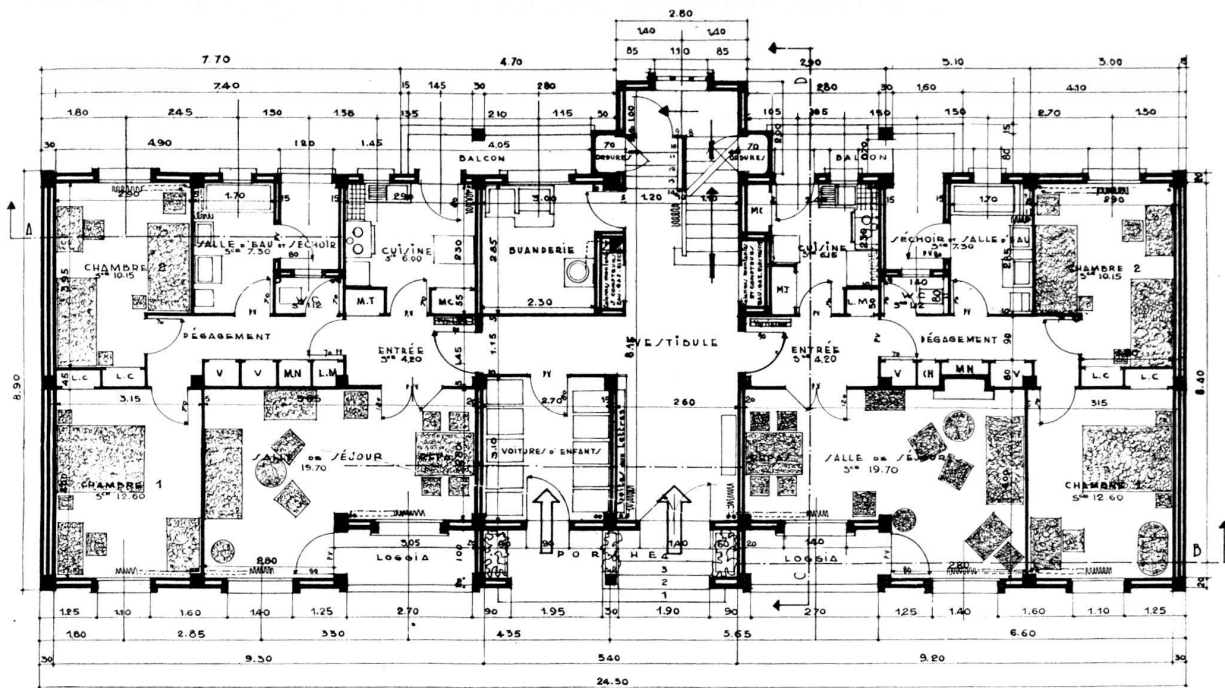
Plan à rez-de-chaussée. Molinié, Sarcé, Chevenot, architectes.
