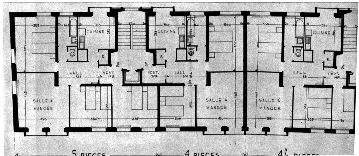
Demi-plan des étages du bloc C.
