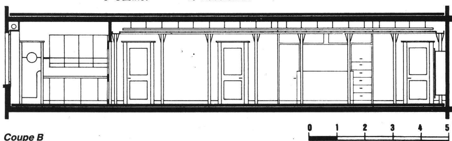
Coupe B
