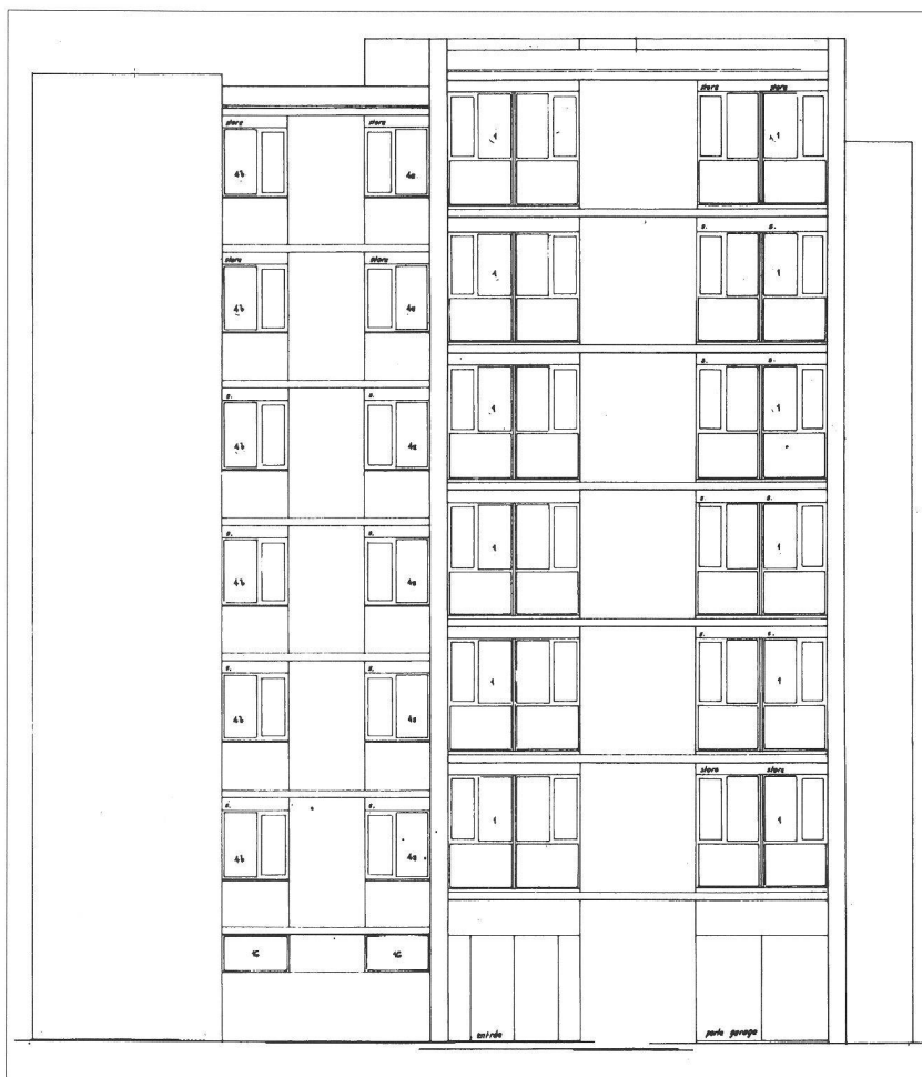
Bâtiment A – façade type (Archives JB + AA)
