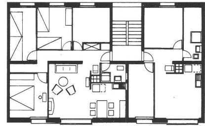
Travée intermédiaire du projet de Georges Addor pour le Concours pour la construction de logements destinés aux «économiquement faibles», Genève, 1952 (dessin de Davide Villa)
