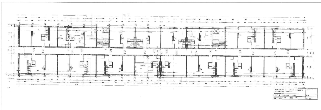
Ci-dessous, le bâtiment D – plan de l'étage-type (Archives JB + AA)
