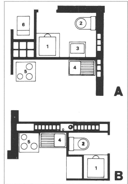
Les «noyaux durs techniques» A – projet de concours de 1952 B – Immeubles C et D 1 – Bain Polyban, servant de baignoire, douche, lavabo et auge à linge 2 – WC 3 – Lavabo 4 – Evier 5 – Fourneau 6 – Poêle (dessin de Davide Villa)
