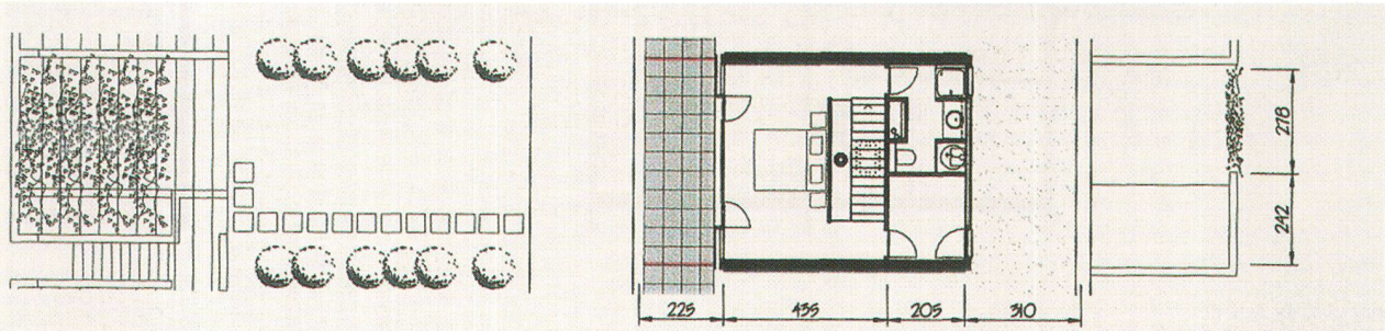
Plan atique
