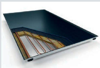
Coupe du nouveau panneau UltraSol de Hoval.
