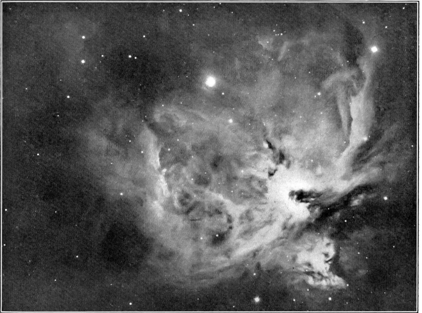
Der große Orion-Nebel. Dreistündige Aufnahme der Mt. Wilson-Sternwarte mit einem Spiegel von 260 cm Öffnung. Der Orion-Nebel ist der einzige sehr helle Gasnebel, der schon mit geringen optischen Hilfsmitteln gesehen werden kann.
