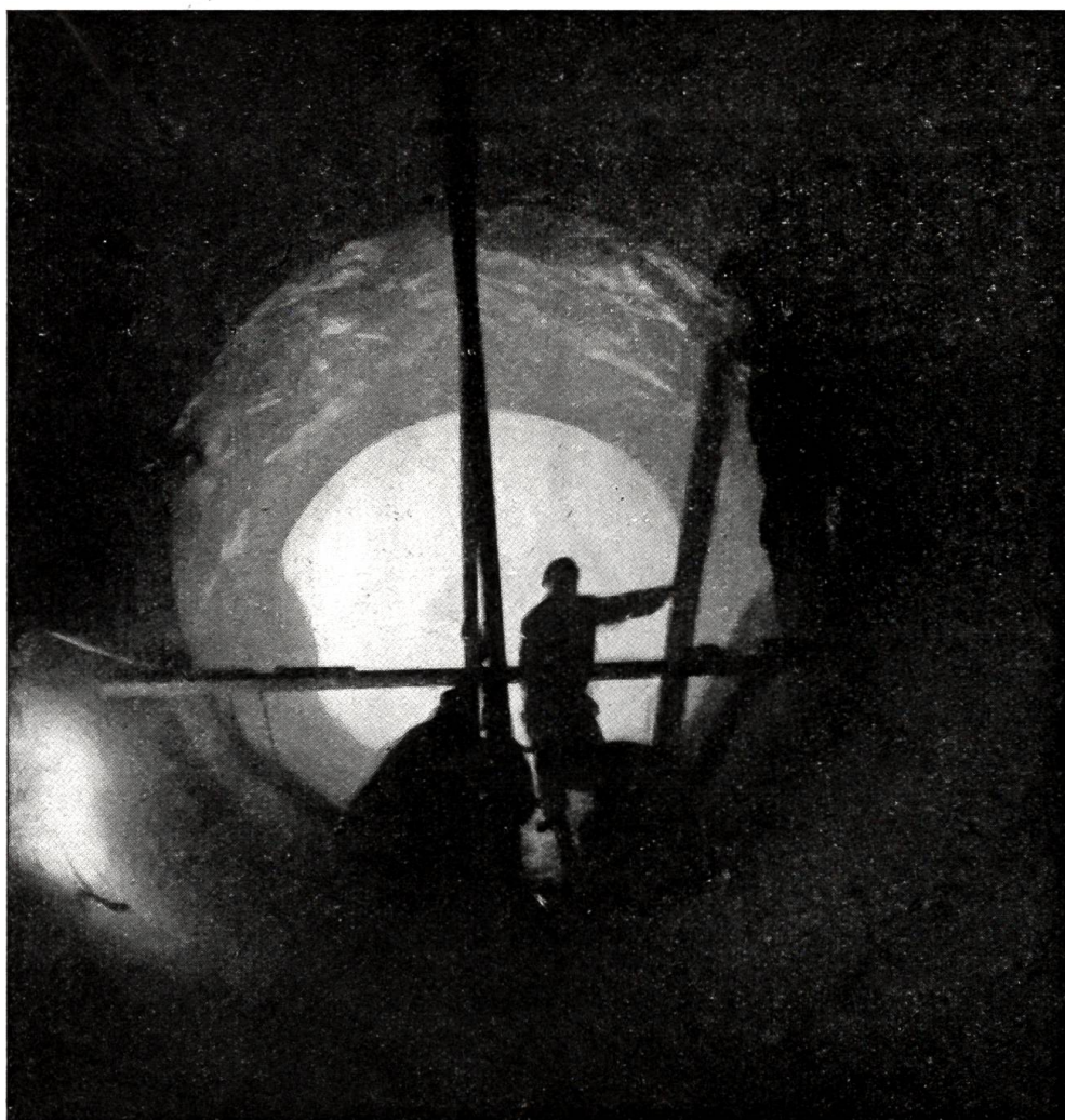
Über 30 km Druckstollenrohre kamen zur Verwendung beim unterirdischen Kraftwerk Innertkirchen. Arbeiter am Schweißen im Bergesinnern.
