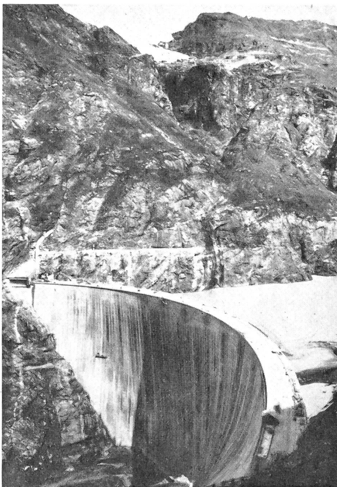
Im Herbst 1958 konnte die Mauvoisin-Staumauer eingeweiht werden. Sie ist 520 Meter lang, 237 Meter hoch und am Scheitel 14 Meter breit.
