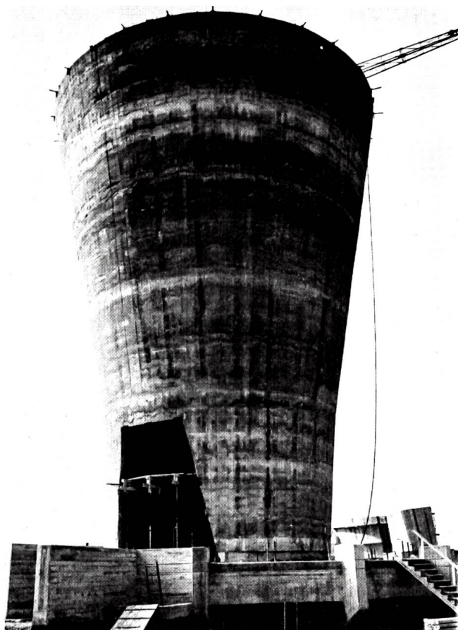
Ein riesiger Kelch in Gimmiz-Walperswil BE Kein Kühlturm eines Atomkraftwerkes, sondern ein 25 m hohes Wasserreservoir in neuartiger Kelchform Photopress-Bilderdienst, Zürich
