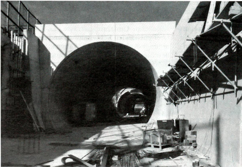
Grossbaustelle Grauholztunnel der SBB
