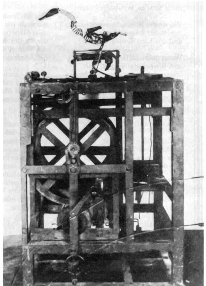
Einblick in den Mechanismus der Ente Seile, die über verschiedene Radtrommeln laufen, bewegen Hebel, die ihrerseits die Ente in Bewegung setzen.
