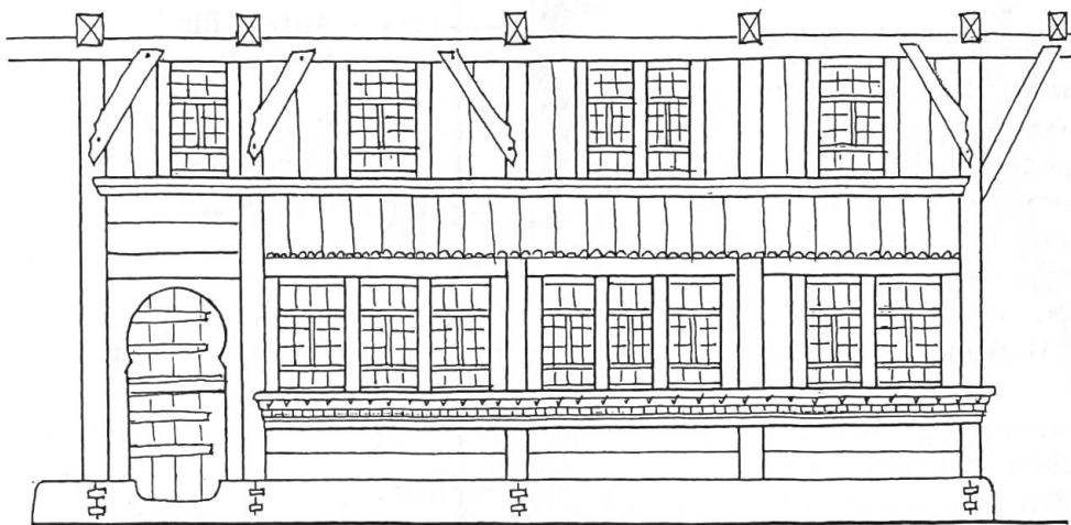
Hochstudhaus Niederönz, Längswand mit Hochstuden
