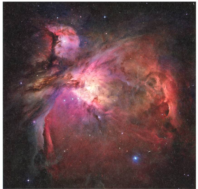
Der Orionnebel ist eine Sternentstehungswolke in rund 1500 Lichtjahren Distanz. Im hellen Zentrum sind mehrere neu entstandene Sterne zu sehen.
