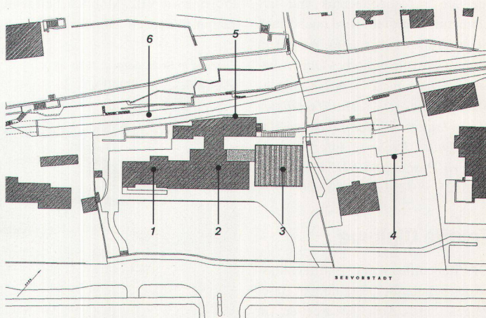
Centre Pasqu'Art, Situationsplan: 1 Altersheim 2 Altes Spital / Centre Pasqu'Art 3 Erweiterungsbau Diener & Diener 4 Mögliche zweite Etappe 5 Nebengebäude mit Filmpodium 6 SBB-Linie Biel-Sonceboz
