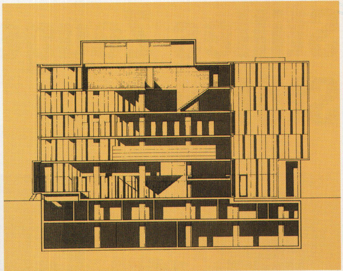
Querschnitt durch den Neubau der Firma Musik Hug von Knapkiewicz und Fickert
