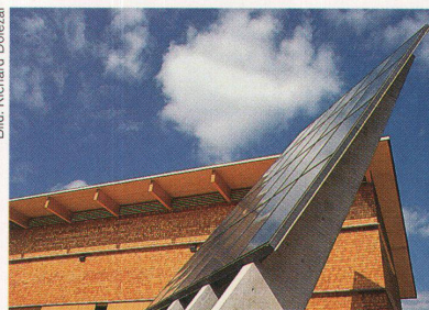
Der freistehende Solarkollektor von Richard Dolezal in Adliswil
