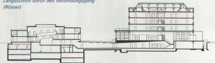
Längsschnitt durch den Verbindungsgang (Rüssel)
