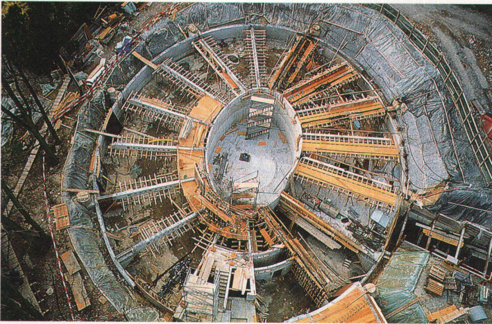
Die Baustelle des Neubaus. Die Betonschraube erreicht die Erdoberfläche
