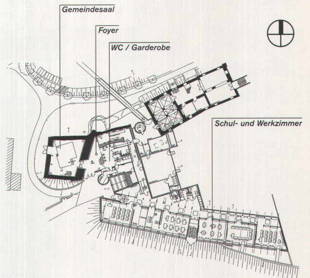
1. Untergeschoss
