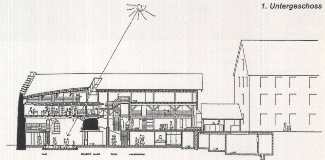
Längsschnitt durch die Trotte
