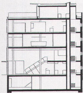
Schnitt durch das zweistöckige Café
