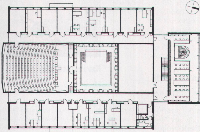
Grundriss zweites Obergeschoss
