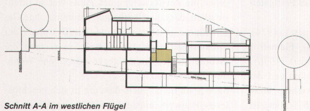
Schnitt A-A im westlichen Flügel
