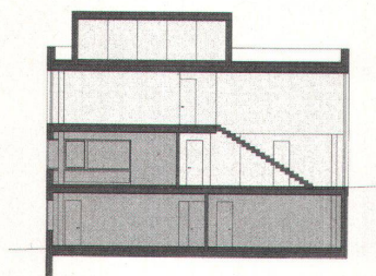
Querschnitt
