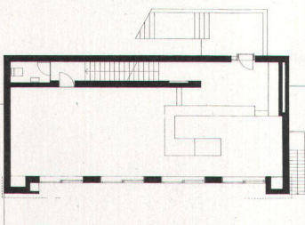
Grundriss Erdgeschoss
