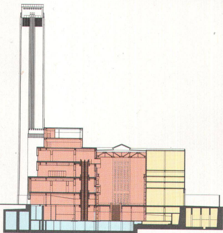
Querschnitt A-A: links das Theaterufer. Die Halle noch mit der ursprünglichen Dachkonstruktion
