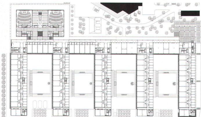
Grundriss eines Normalgeschosses
