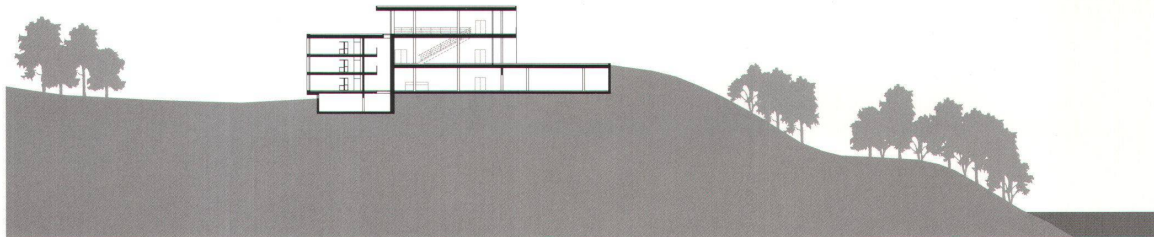
Querschnitt im mittleren Bereich. Das Gebäude steht hinter der Krete und nützt die Senke der Mulde für einen Split-Level-Schnitt aus. Unter der Terrasse liegt die Tiefgarage.
