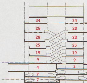
Querschnitt A-A
