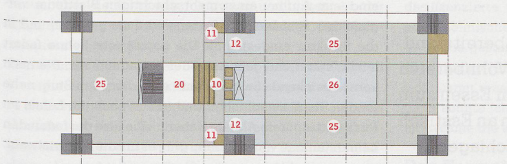
2. OG, Seminarageschoss
