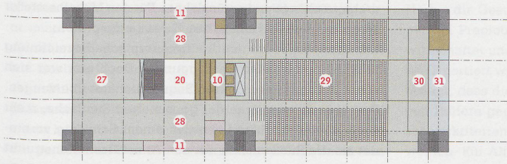
3. OG, Kongressgeschoss
