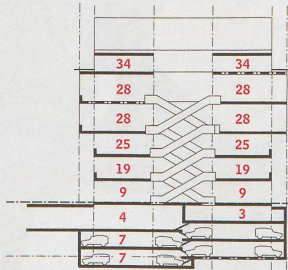
Querschnitt A-A
