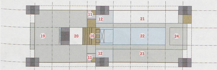
1. OG, Verwaltungsgeschoss
