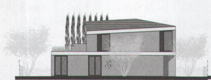
Nordwest Fassade
