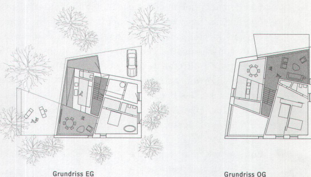
Grundriss EG
