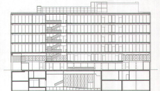
Schnitt
