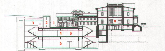
Längsschnitt
