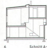
6 Schnitt A-A
