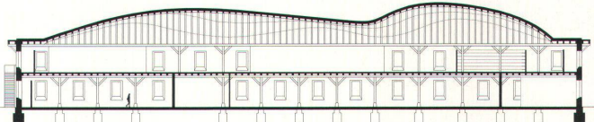
^ Längsschnitt durch das Oberlicht
