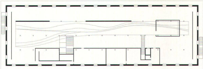
^ Grundriss Obergeschoss
