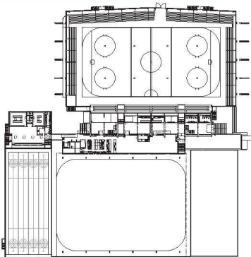
^45_ Eiszentrum, Grundriss.
