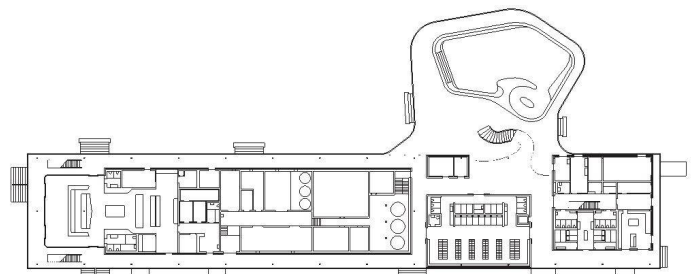
^Grundriss Erdgeschoss
