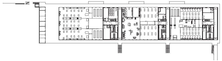
∨ Obergeschoss: Über den Kernen liegen jeweils zwei Klassenzimmer.
