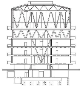
^ Querschnitt: Hort und Mensa im Erdgeschoss, drei Geschosse Klassenzimmer, Lehrerzimmer, Bibliothek und Turnhalle auf dem Dach.
