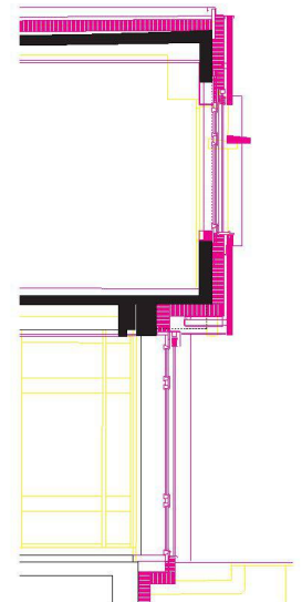
✓Fassadenschnitt Spezialtrakt: Die Betonelemente sind aufgehängt.
