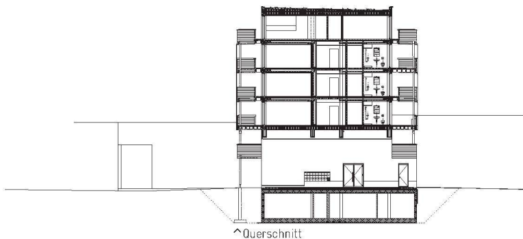
^Querschnitt
