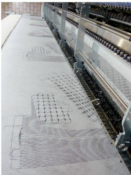
Versuch in der Produktionshalle von Forster Rohner: Die Stickmaschine bringt Sensoren auf Textilien.
