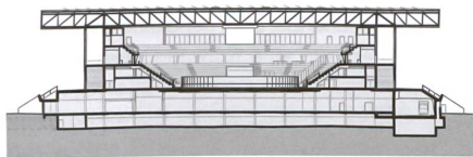
Querschnitt Eishockeystadion. 0 25 50 m
